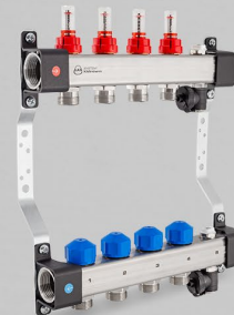
Kollektor vooluhulgamõõturite, ajamiga ventiilide ja õhueraldiga, seeria N75A
