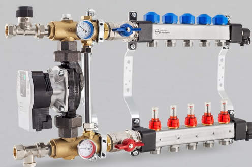
Kollektor vooluhulgamõõturite, ajamiga ventiilide ja elektroonilise juhtimisega pumbaga segamissõlmega, seeria N77E
