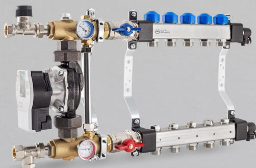
Kollektor reguleeriventiilide, ajamiga ventiilide ja elektroonilise juhtimisega pumbaga segamissõlmega, seeria N73E
